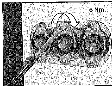
Фигура 4.29: Затягане на тапите
