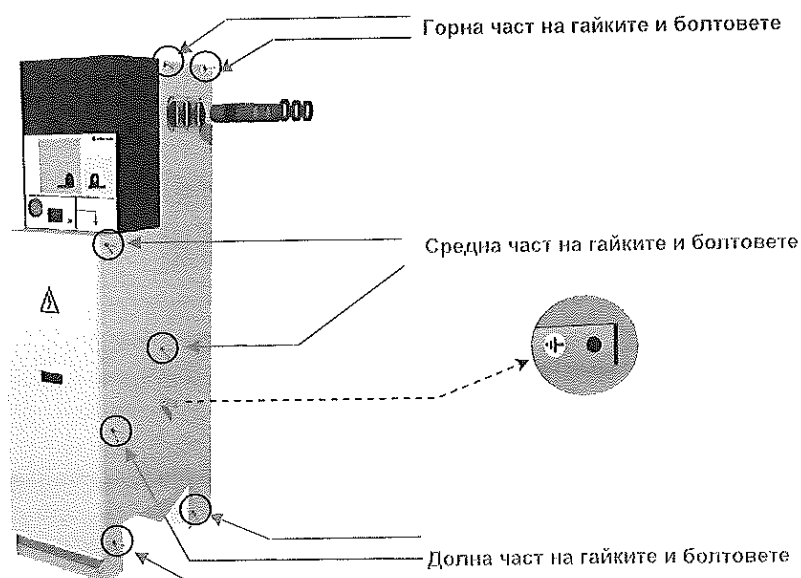
Фигура 4.21: Подробен изглед на точките за салобяване на гайките и болтовете
