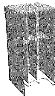
Фигура 5.14: Подробен изглед на клемната кутия
