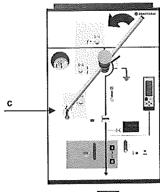
Фигура 5.47: Процес по завъртане на лоста
