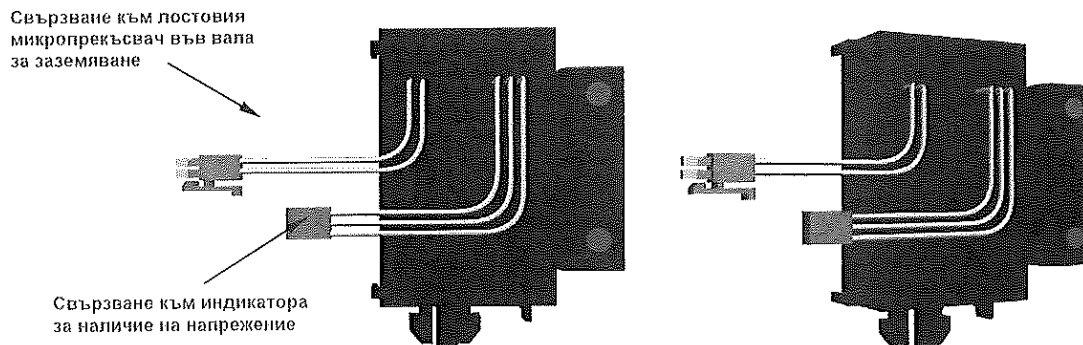
Фигура 6.4: Свързване на ekorSAS
