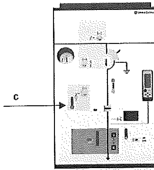
Фигура 5.59: "Готов за заземяване" шкаф за прекъсвачи
